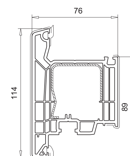
103.386 außen öffnend Verstärkung 113.270, 113.368.2, 115.003
