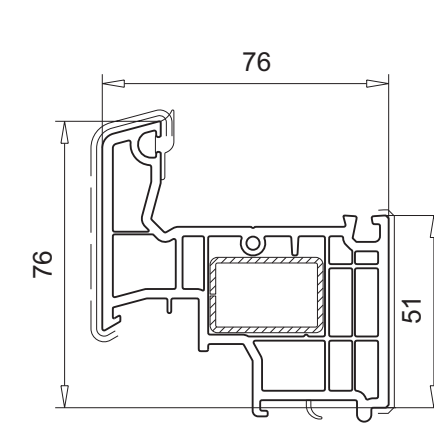
103.384 Aufbauprofil für Flügel 84 mm Verstärkung 113.019
