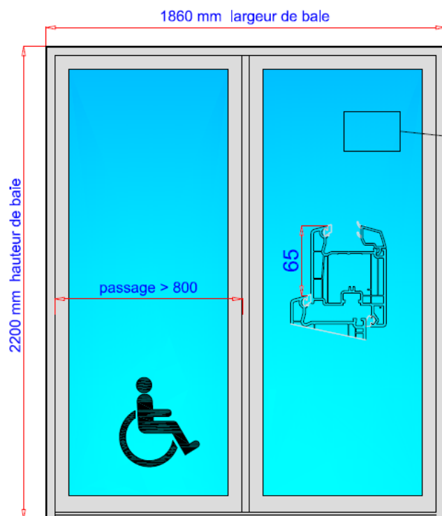
Porte-fenêtre standard (ouvrant porte-fenêtre serrure)
