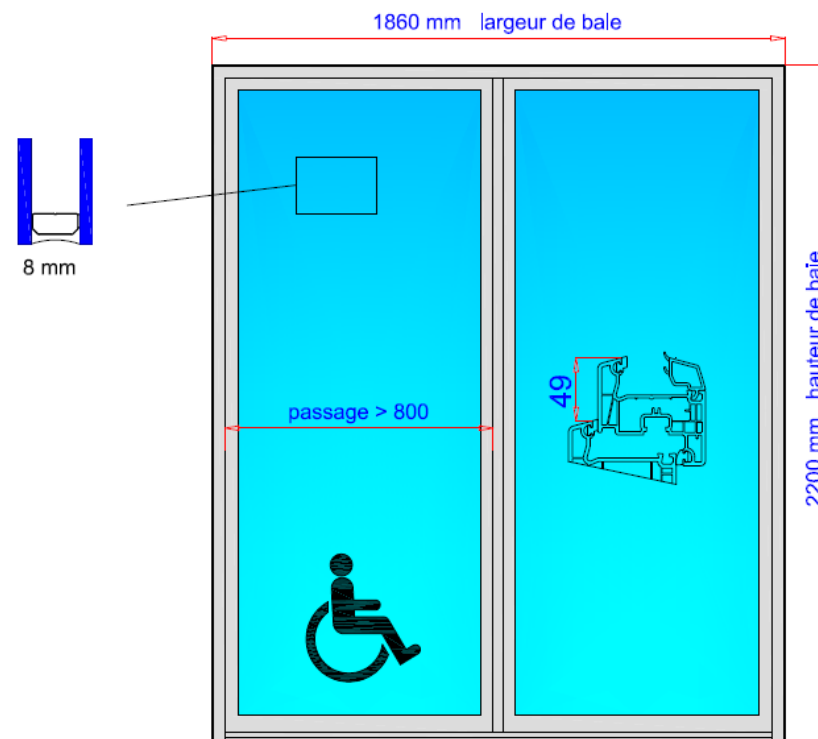
Porte-fenêtre Vision XXL (le plus petit ouvrant)
