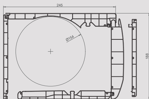
Kit coffre 188 119.605 avec trappe arrondie 119.606 avec trappe droite
