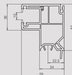
Coulisse pour lame M37 108.114
