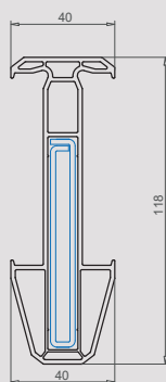
Accouplement 118 x 40 mm 116.207
