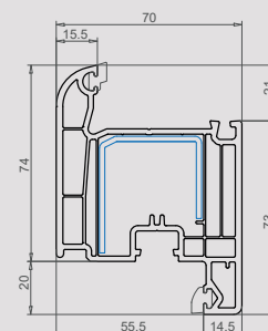
Ouvrant serrure 94 mm 103.289
