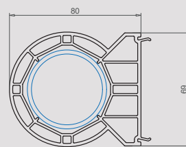
Accouplement d'angle variable 116.206
