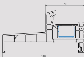
Dormant 74 x 146 mm Isolation de 140 mm 101.267
