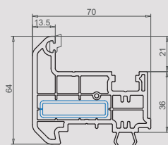
Battement rapporté 64 mm 102.234
