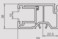
Coulisse pour lame M37 108.112
