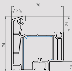
Battement monobloc 74 mm 103.318
