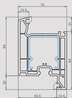
Ouvrant intérieur 105 mm 103.241
