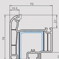
Battement monobloc 74 mm 103.288
