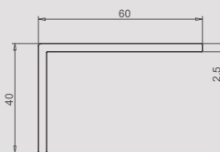
Cornière 40 x 60 mm 109.001
