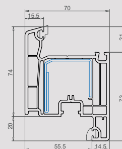
Ouvrant serrure 94 mm 103.357
