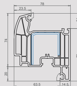
Ouvrant serrure 94 mm 103.333
