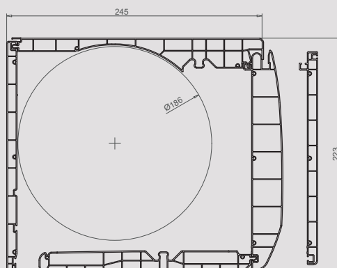
Kit coffre 223 119.603 avec trappe arrondie 119.604 avec trappe droite
