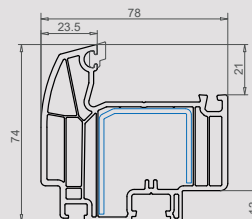
Battement monobloc 74 mm 103.332
