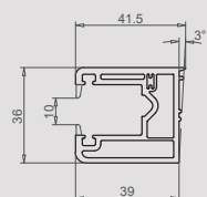
Coulisse pour lame M37 108.113
