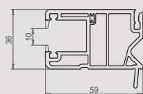
Coulisse pour lame M37 108.111
