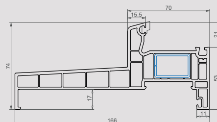
Dormant 74 x 166 mm Isolation de 160 mm 101.244
