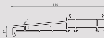
Pièce d'appui 70 mm 110.080
