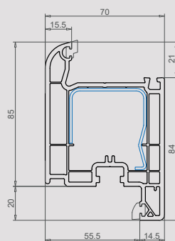
Ouvrant intérieur 105 mm 103.273
