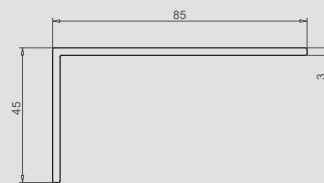
Cornière 45 x 85 mm 109.134
